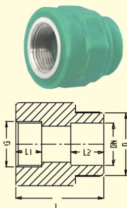
NÓI RĂNG TRONG (Female Threaded Coupling)
